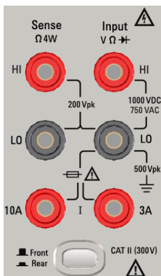
34461A, 34465A, 34470A: Лицевая панель Область разъемов
