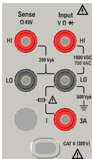
34460A: Лицевая панель Область разъемов
