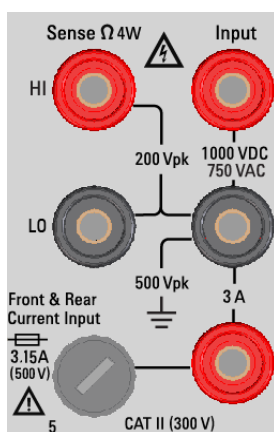
34461A, 34465A, 34470A: Задняя панель Область разъемов
